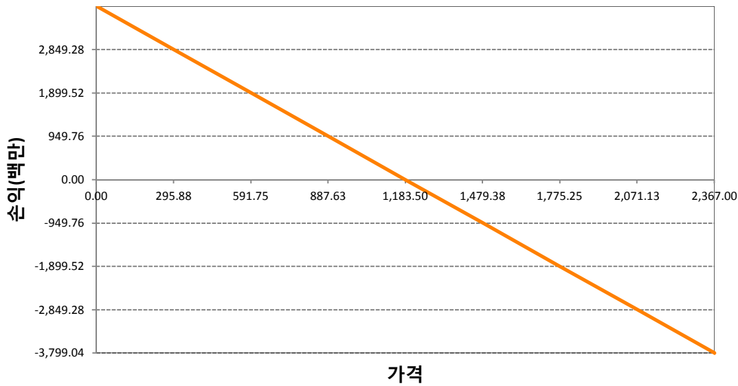
KR4175Q90003-2020-09 달러선물
