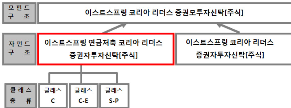
[집합투자기구의 구조]
